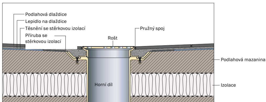
Detail těsnění s tenkým ložem
