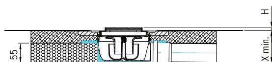
Systémová deska s odtokovým tělesem DN 50, spád 1,5°, zápachový uzávěr 30 mm, spodní prvek 55 mm
