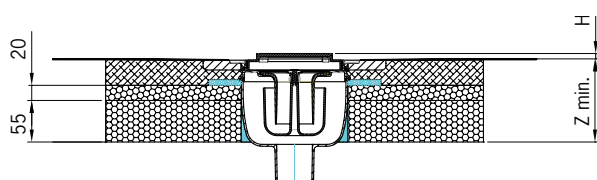
Systémová deska s odtokovým tělesem DN 50, spád 90°, zápachový uzávěr 50 mm, spodní prvky 55 mm + 20 mm
