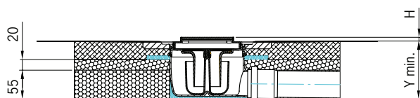
Systémová deska s odtokovým tělesem DN 50, spád 1,5°, zápachový uzávěr 50 mm, spodní prvky 55 mm + 20 mm
